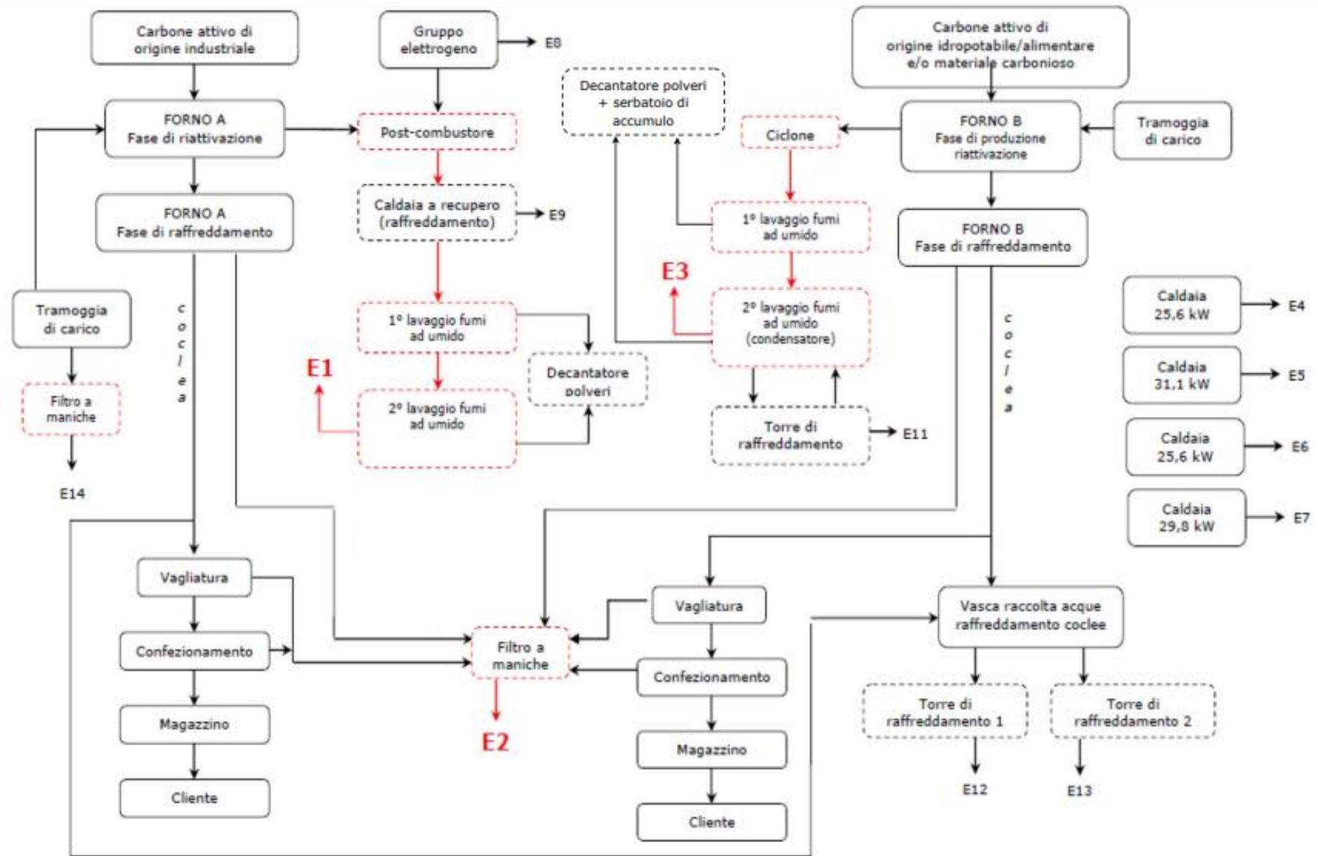
Figura 12 – Ciclo di lavorazione e interazioni ambientali
